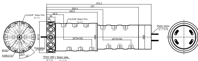
MK123-MT2586 尺寸图 12进12出G3/8"牙+信号(5A、10A)
